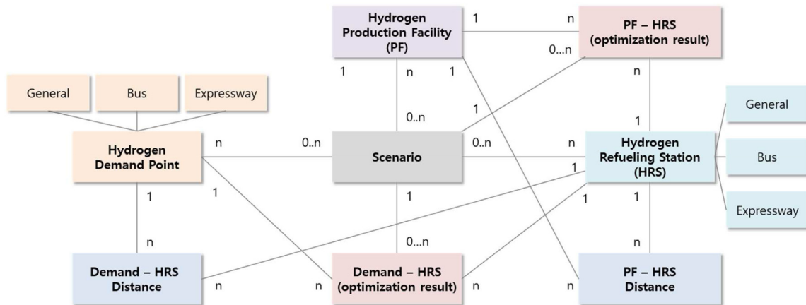
Fig. 5 – Data model.
